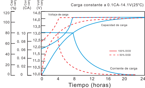
Curva de Carga
